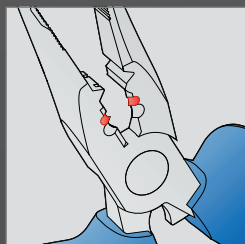
Snímanie izolácie od \varnothing 2,2 mm do \varnothing 3,0 mm.
