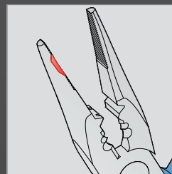
Ohýbanie tvrdého drôtu a výroba očiek do \varnothing 3,5 mm. Zárezy na oboch stranách čelustí.
